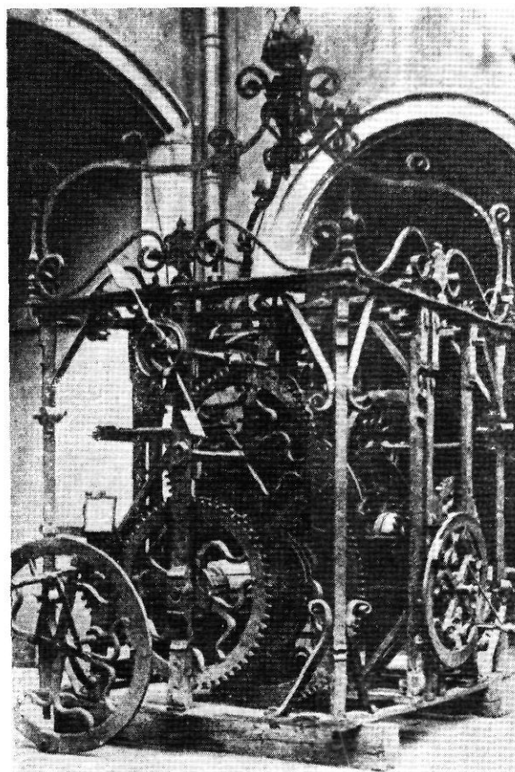
Maquinària del rellotge de la torre de la Catedral de Barcelona. (Foto "Gran Enciclopèdia Catalana").
